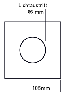
Gehäuseoberteil viereckig
