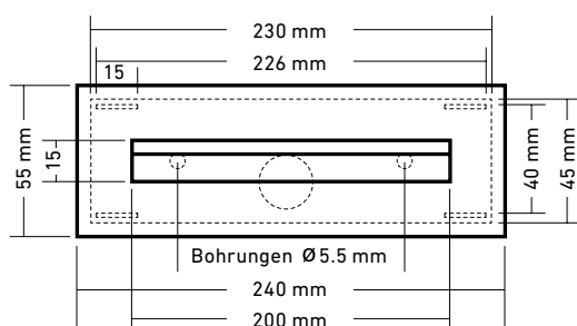
Down Light 200, Frontansicht
