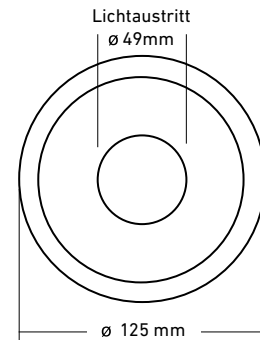
Gehäuseoberteil gross
