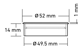
Montagehülse
