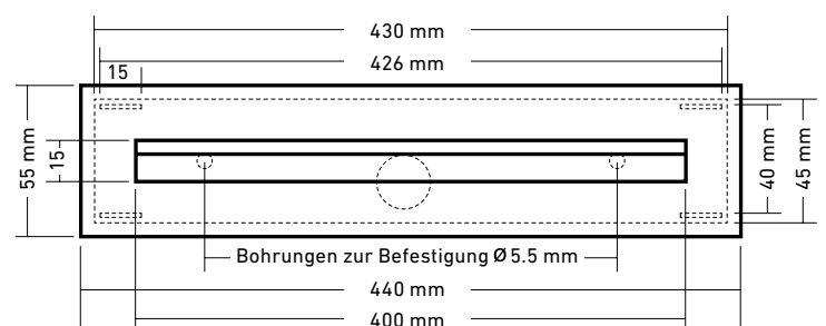
Down Light 400, Frontansicht
