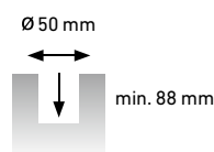
Montagehülse
