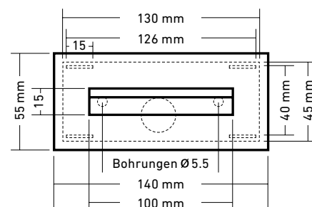
Down Light 100, Frontansicht
