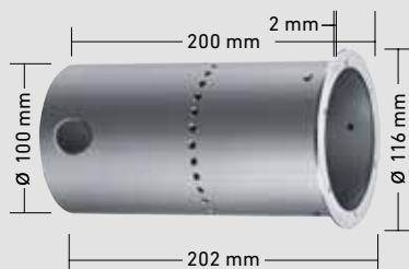
Montagerohr Wabenspot
